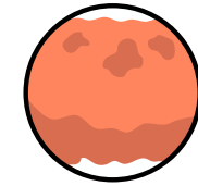
Mars
